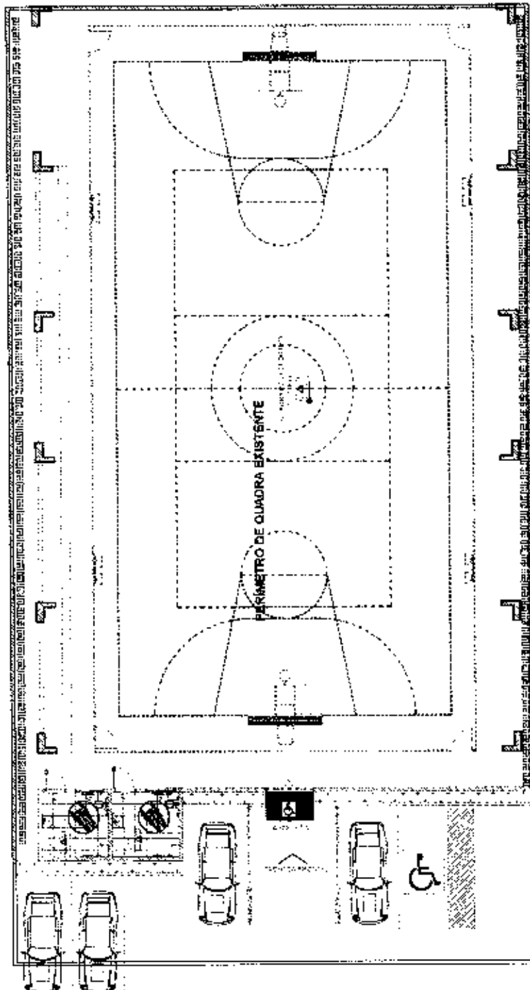
PLANTA BAIXA DE CONSTRUÇÃO E IMPLANTAÇÃO
